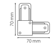
соединитель однофазный BARRA L-образный
