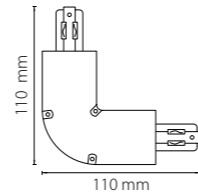
соединитель трехфазный BARRA L-образный
